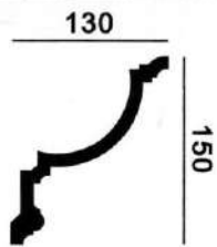
A088- 4”/5”
